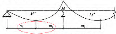
图 14.3.4 连续梁剪跨区划分图
