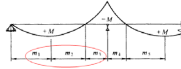
图 11.3.4 连续梁剪跨区划分图
